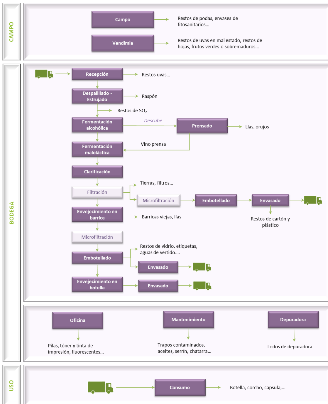
Figura 2. Diagrama de flujo de producción del vino.
