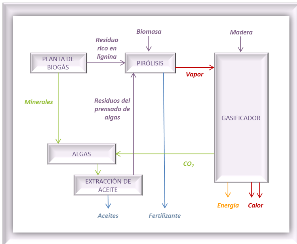
Figura 7. Proceso propuesto en el proyecto ICON power.
