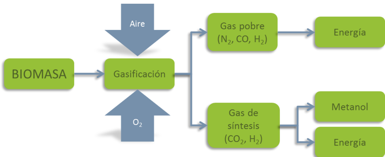
Figura 6. Proceso de gasificación para obtención de metanol
