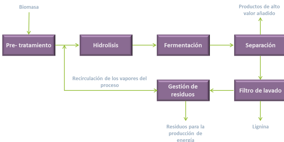
Figura 5. Proceso de obtención de bioetanol a partir de residuos lignocelulosicos.
